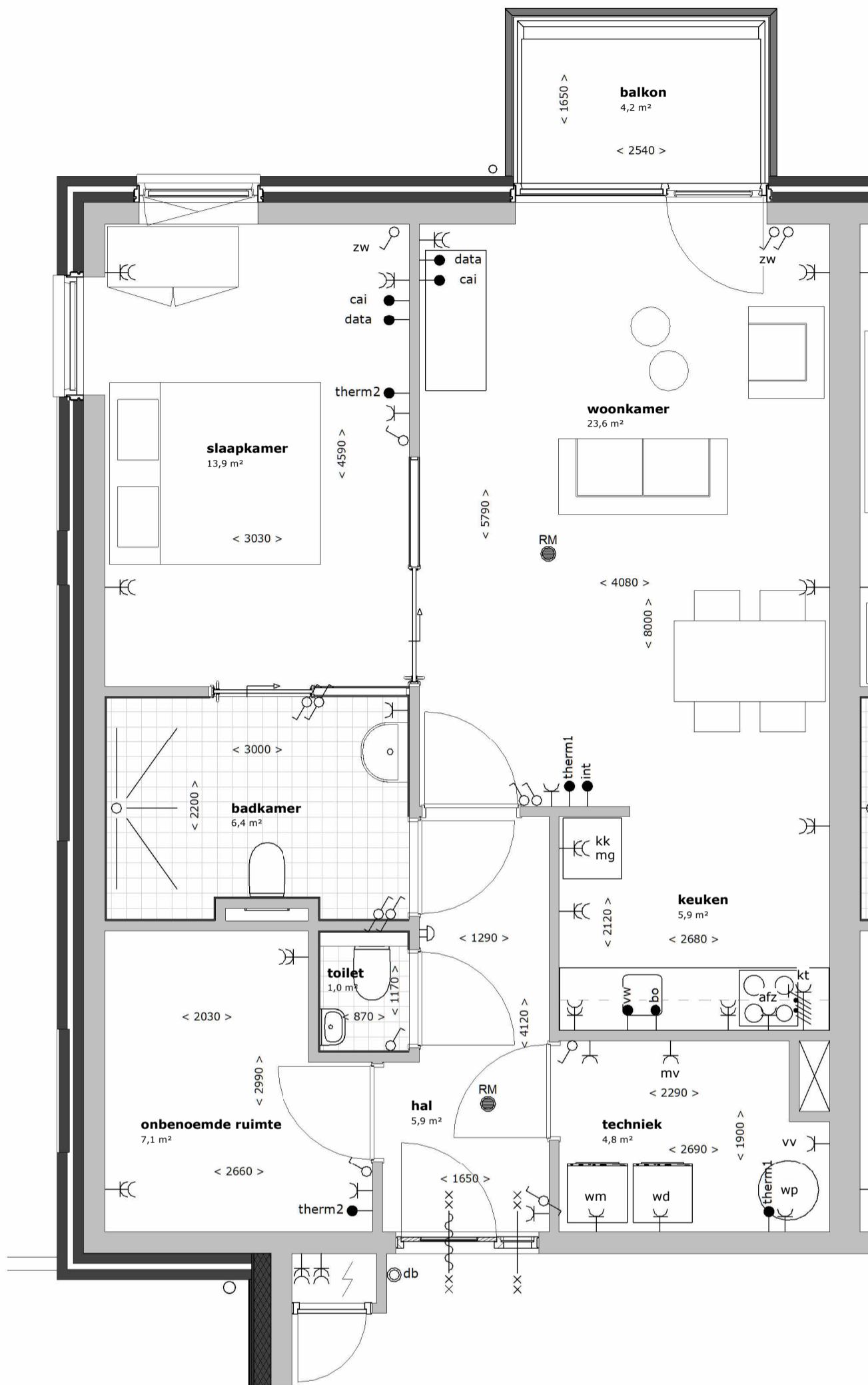
appartement type B6
