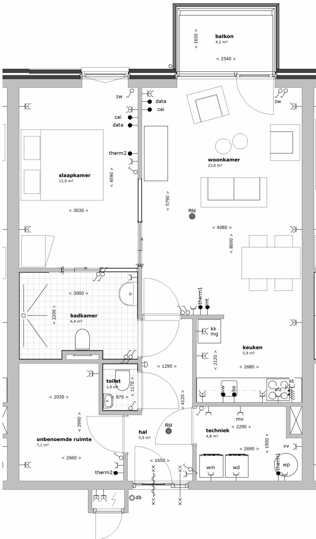
appartement type B5
